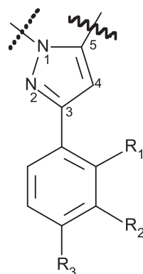
Pyrazol-1,5-diyl
