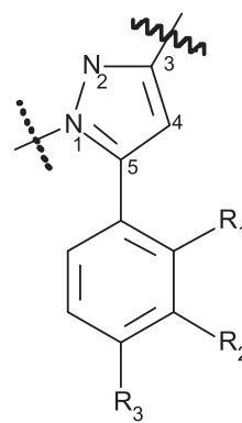
Pyrazol-1,3-diyl
