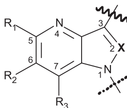
4-Aza-Derivate
